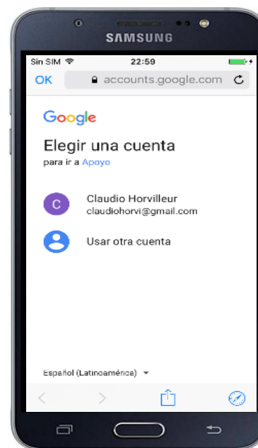
Figura 59. Autenticación Google
