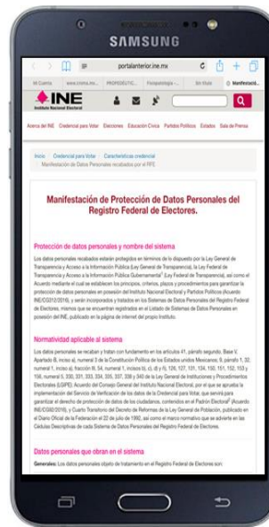
Figura 38. Más información.
